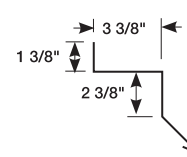
7/8" J TRIM
